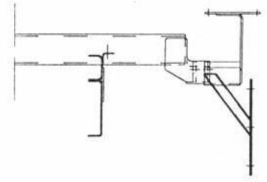
Ansicht Y
